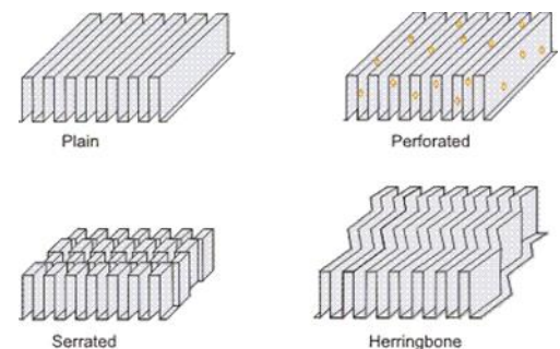
Bild2: mögliche Rippenvariationen
