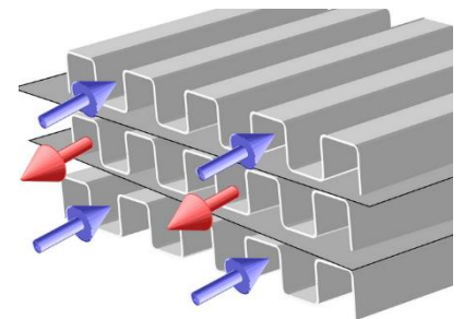
Bild1: Schema eines PFHE mit zwei kalten und einer warmen Platte
